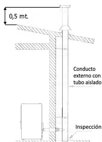
Fig. 3: conexión a un conducto exterior con tubo aislado o doble pared una cumbreira antiviento
