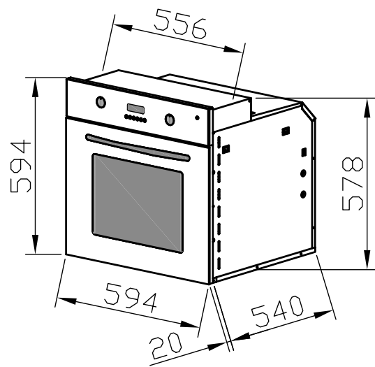
Figura 3. Dimensiones del horno
