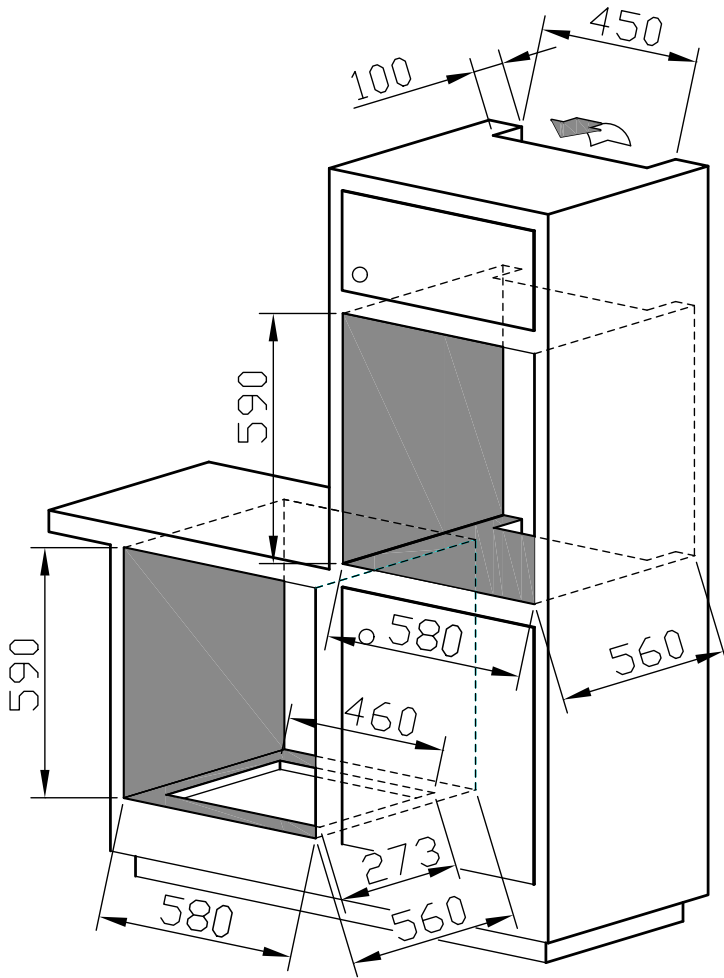
Figura 4. Dimensiones del gabinete
