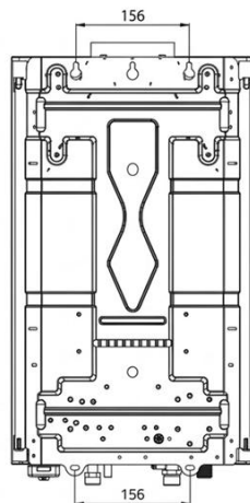
Dimensiones Instalación
