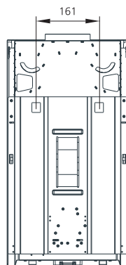
Dimensiones Instalación
